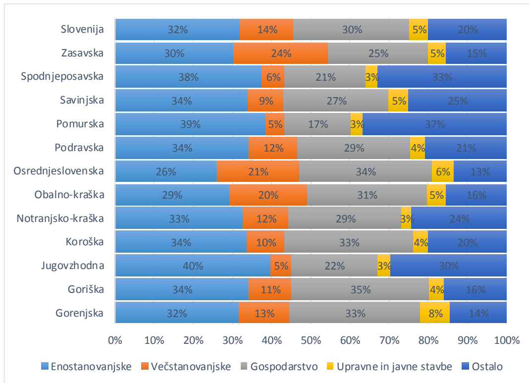
Slika 5: Delež površine streh glede na namenskost stavb za statistične regije
