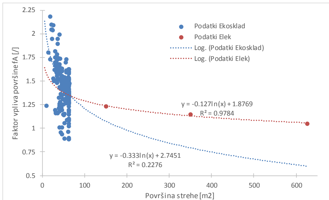
Slika 27: Določitev faktorja vpliva površine f_A
