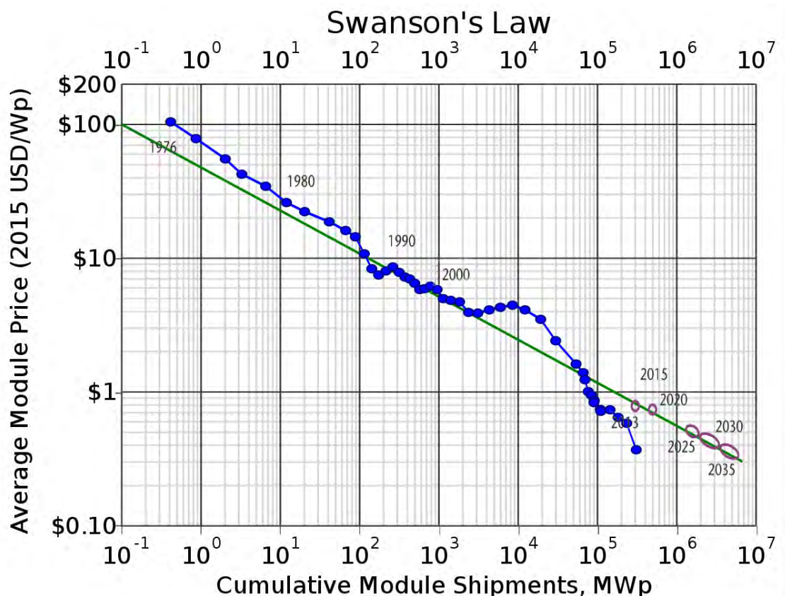
Slika 24: Swansonov zakon: padajoče cene panelov v odvisnosti od količine letne proizvodnje
