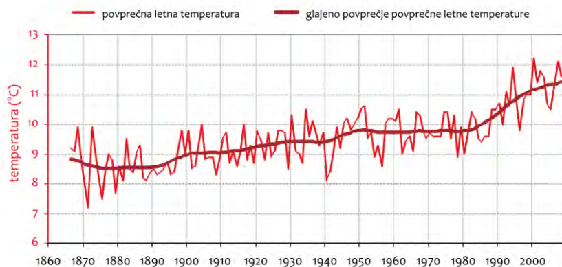
Slika 10: Povprečna temperatura v Ljubljani (48)
